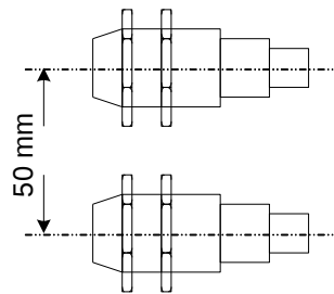
Bild 2 Gegenseitige Beeinflussung
