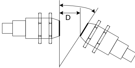
Bild 4 Winkelversatz
