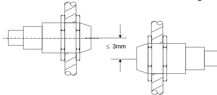
Bild 5 Seitenversatz
