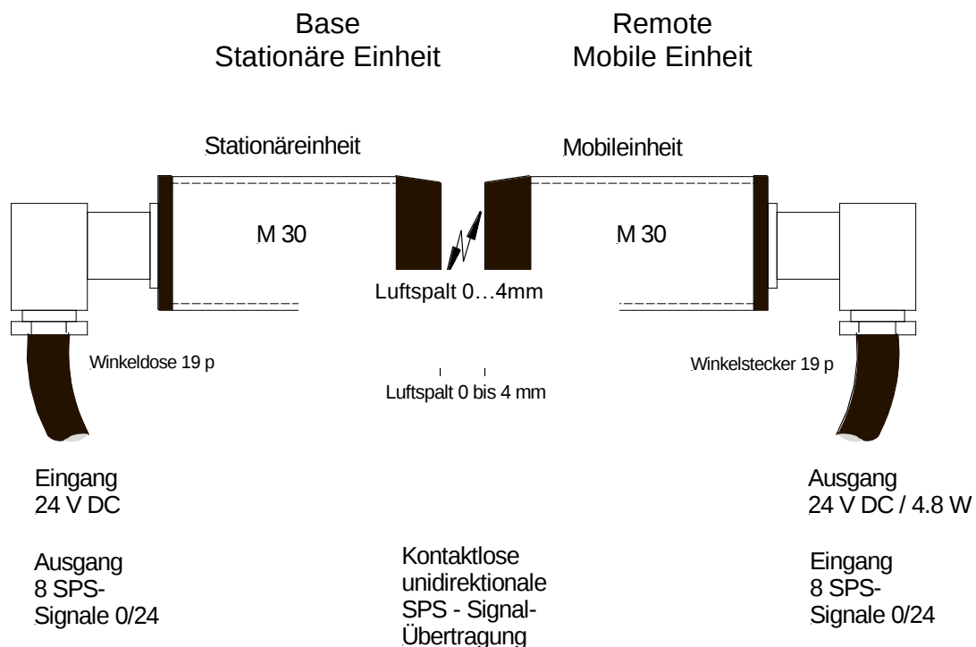
Bild 6 Übertragungskette
