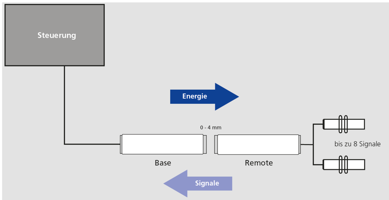
Bild 1 Funktion induktives Übertragungssystem Gamma Simplex
