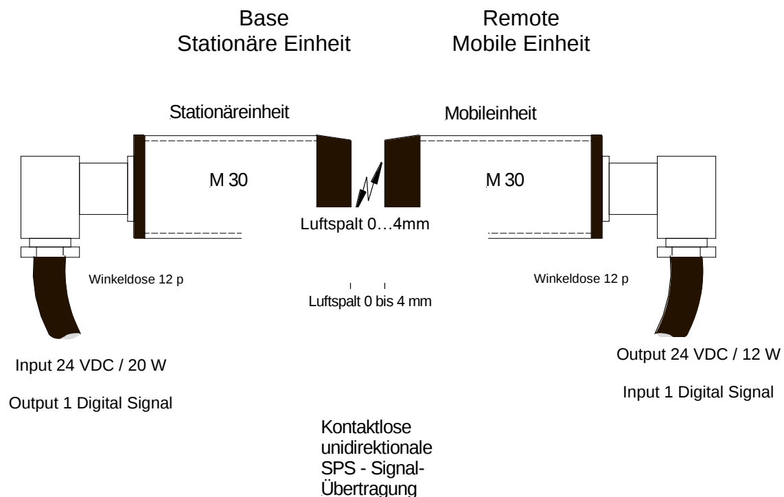
Bild 6 Übertragungskette
