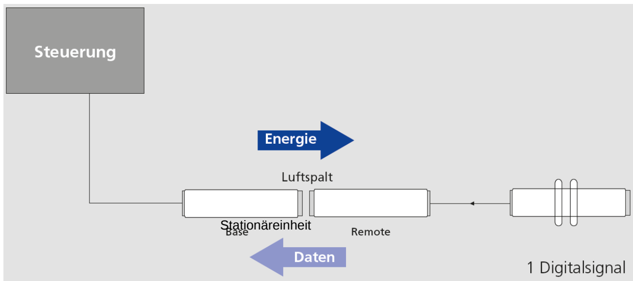
Bild 1 Funktion induktives Übertragungssystem
